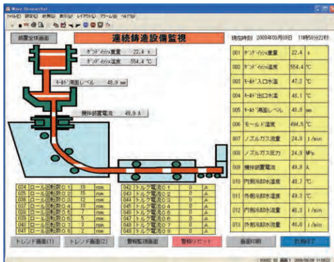
連続鋳造設備全体図表示例
